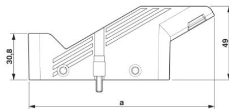
Rozměrový výkres, a=123,7
