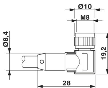
Zdíčka M8 x 1, úhlová, s LED diodami
