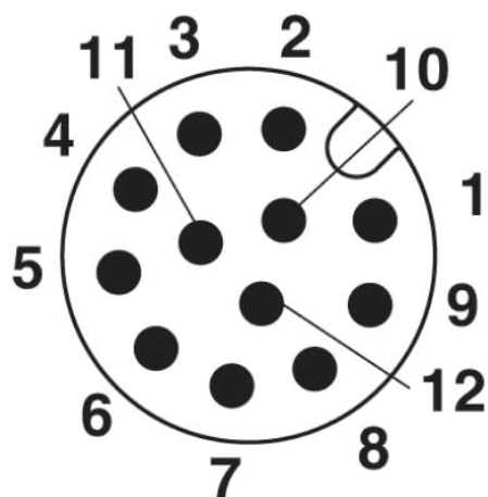
Obsazení pólů zástrčky M12, 12pólová, pohled ze strany kolíku
