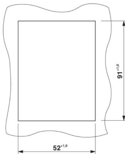
Montážní otvor
