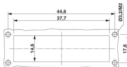
Montážní otvor
