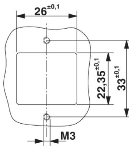
Montážní otvor
