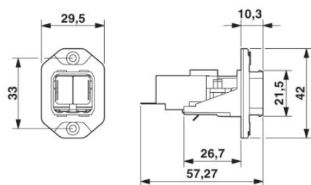
Montážní rám Push-Pull SCRJ
