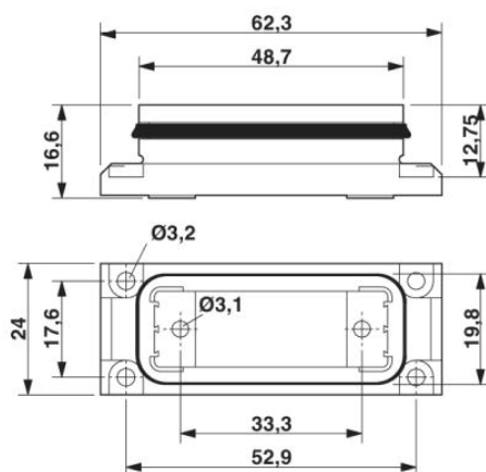
Montážní rám D-SUB
