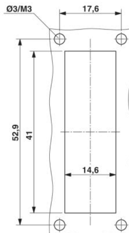
Montážní otvor
