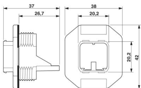
Montážní rám Push-Pull, systém Freenet, IP67
