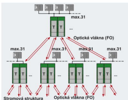
redundantní hvězdicová struktura
