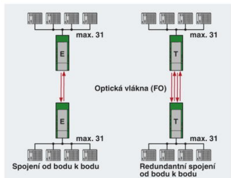
redundantní spojení bod-bod
