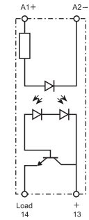
princiální schéma
