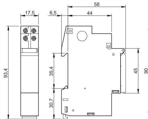
12.22 šroubové svorky
