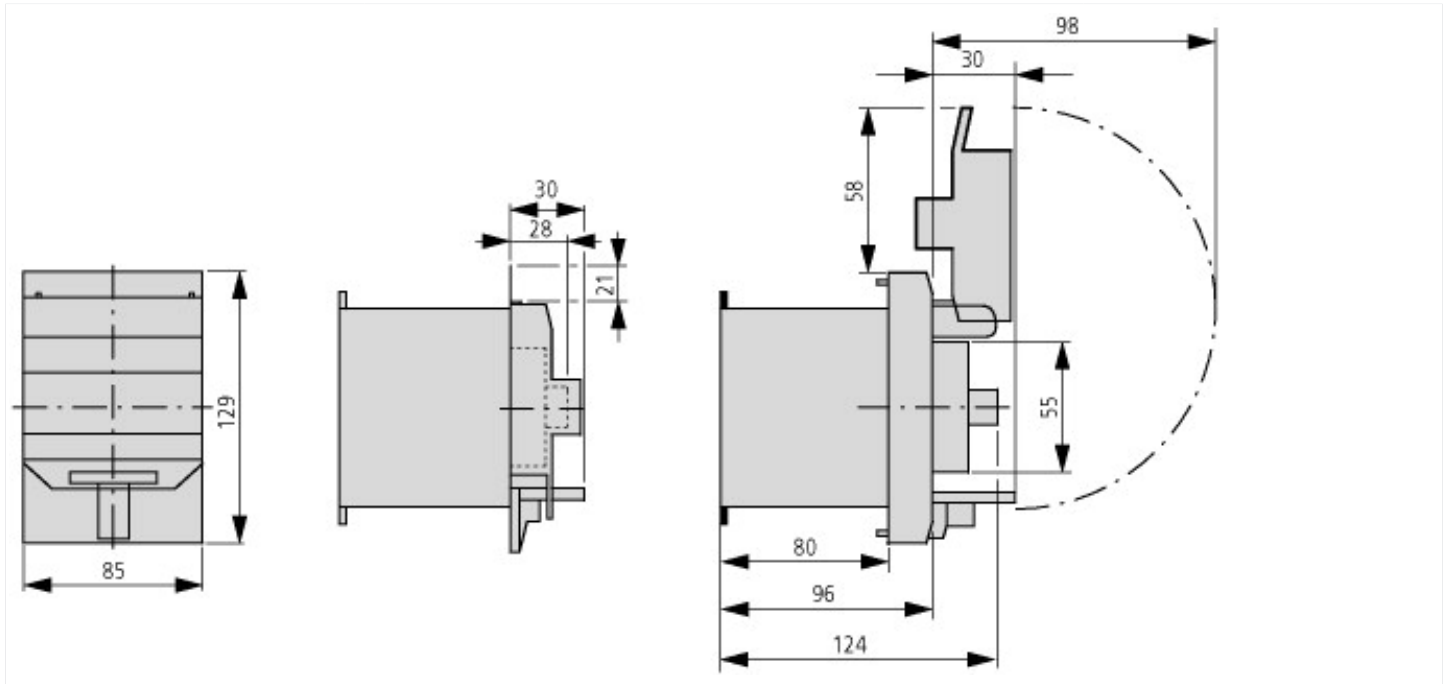
Vestavná skříňka z izolačního materiálu E-PKZ0-G... + SVB-PKZ0-E
