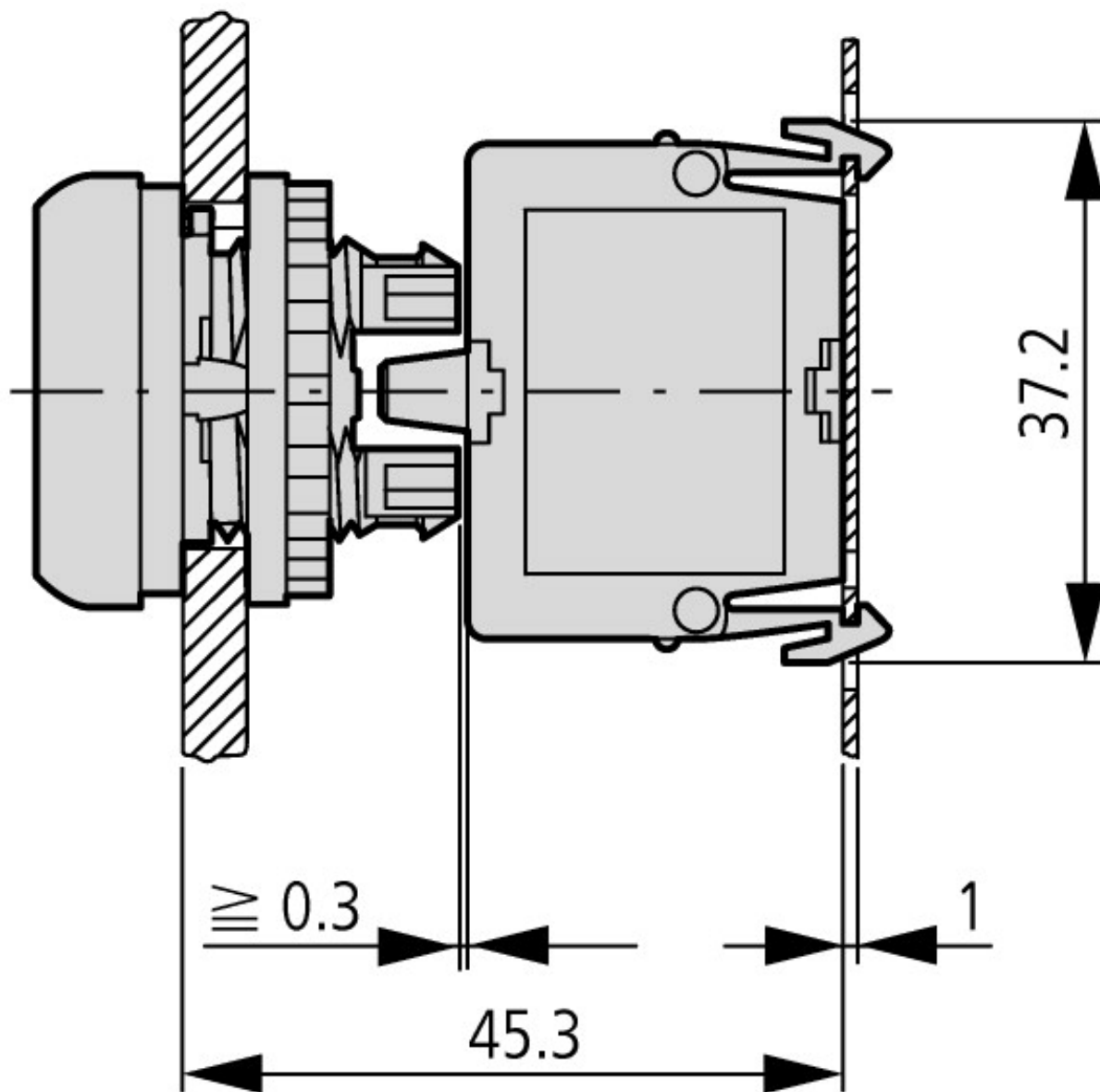
Ovládací a signalizační prvky v zadním upevnění
