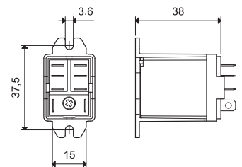
056.25 s relé
