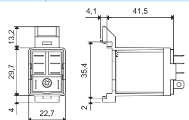
056.27 s relé
