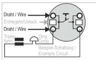
Příklad pro zapojení tlačítka.
