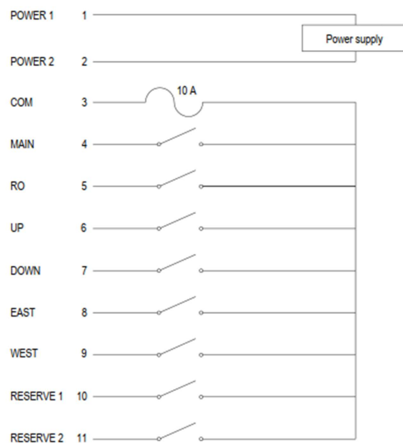
Připojovací schéma (obj. č. 2832830 / 2832831)
