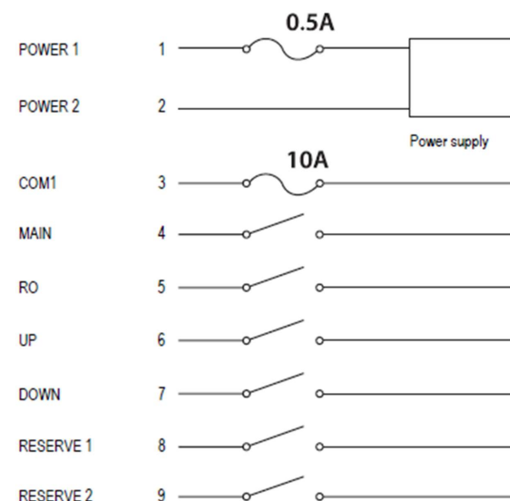
Připojovací schéma (obj. č. 3208797 / 3208798)
