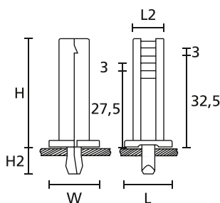
TY5K5 montagesokkel med nitte
