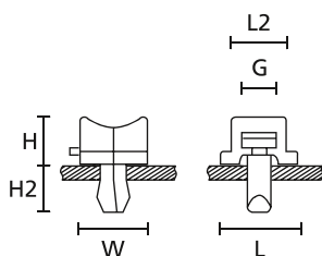
TY5K2 montagesokkel med nitte
