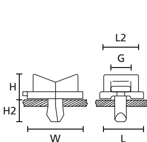
TY5K3/5 montagesokkel med nitte
