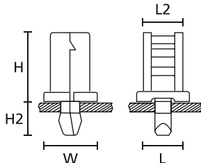
TY5K1 montagesokkel med nitte
