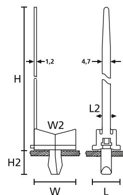
TY5K4 montagesokkel med nitte
