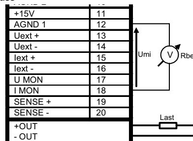
Bild 7.7 Verdrahtung Strommonitor.
