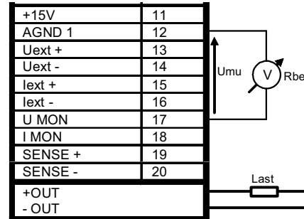
Bild 7.6 Verdrahtung Spannungsmonitor.
