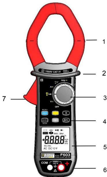
Abbildung 1 : Vielfachmesszange F603
