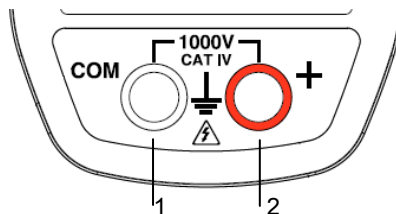
Abbildung 5 : Anschlussbuchsen
