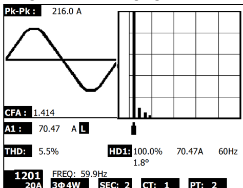
Abbildung 5-7b: Oberschwingung - Bildschirm 2
