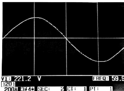
Abbildung 5-9a: Wellenformen - Bildschirm 1
