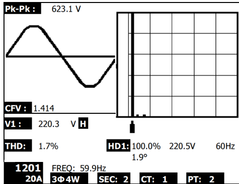
Abbildung 5-7d: Oberschwingung - Bildschirm 4
