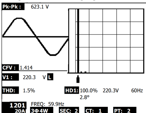
Abbildung 5-7a: Oberschwingung - Bildschirm 1
