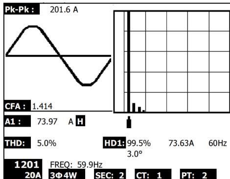
Abbildung 5-7d: Oberschwingung - Bildschirm 4
