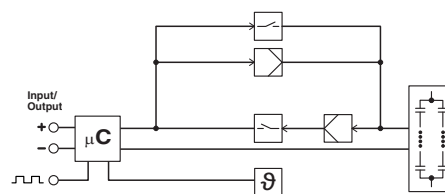
Blockschaltbild
