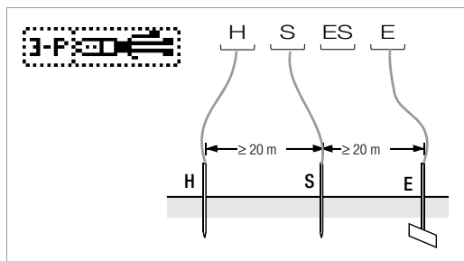
Messung des Erdungswiderstandes nach dem Dreileiterverfahren
