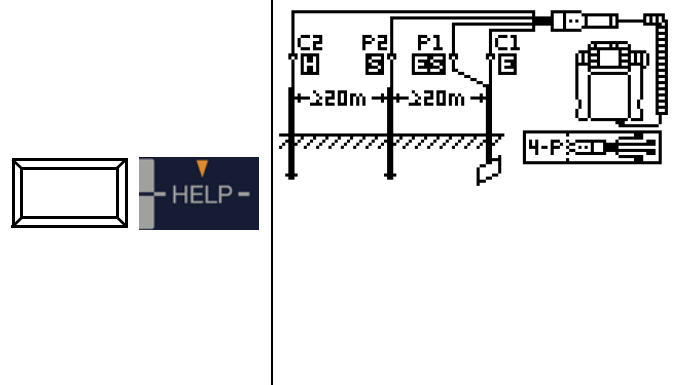
Bild 10.8.1 Messung des Erdungswiderstandes nach dem Vierleiterverfahren
