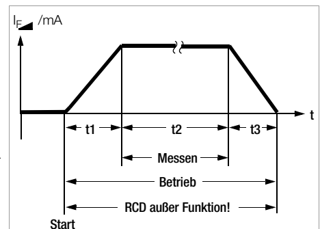
Unterdrückung der RCD-Auslösung bei pulsstromsensitiven RCD-Schutzschaltern
