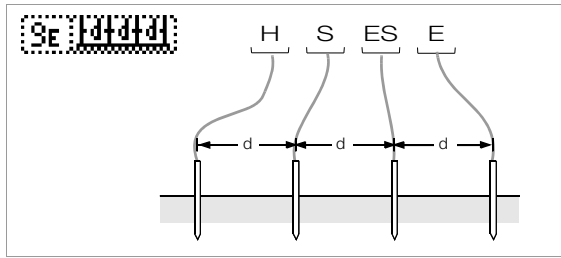
Messung des spezifischen Erdwiderstandes
