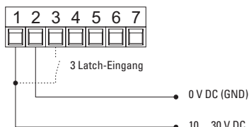
Anschluss Spannungsversorgung und Latch-Eingang
