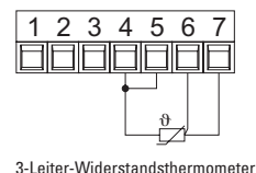
Anschluss Widerstandsthermometer Pt100/Ni100
