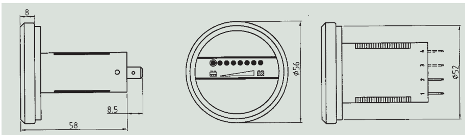
Typ 827, 827.6, 827.7
