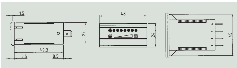
Typ 828, 828.6, 828.7
