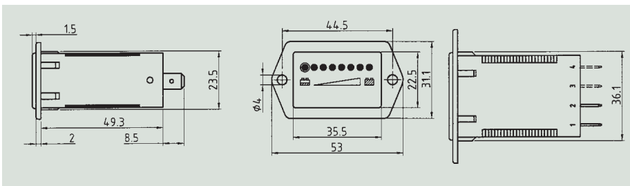
Typ 826, 826.6, 826.7
