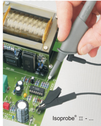
Passiver Tastkopf, hohe Eingangskapazität
