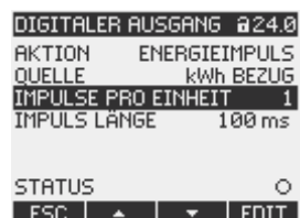
Bild 3-6 Arbeitsimpulsausgang
