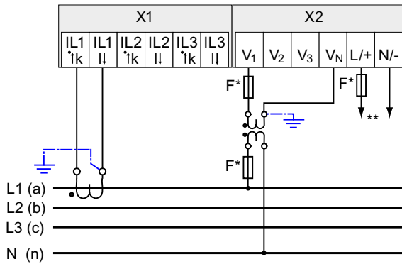
Bild 6-11 Anschlussart 3P4WB, mit Spannungswandler, mit einem Stromwandler
