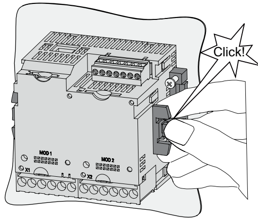
Montageschritt C
