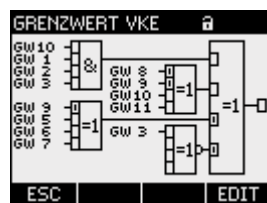
Bild 3-12 GRENZWERT VKE
