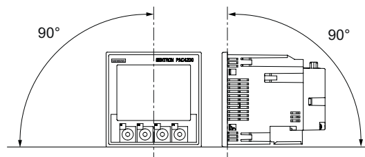
Bild 4-1 Einbaulage
