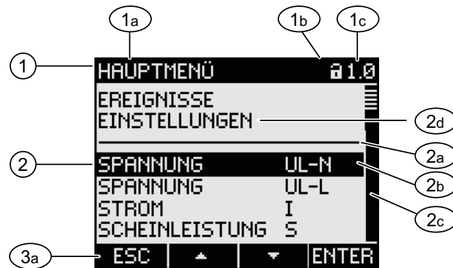
Bild 8-9 Anzeige "HAUPTMENÜ"
