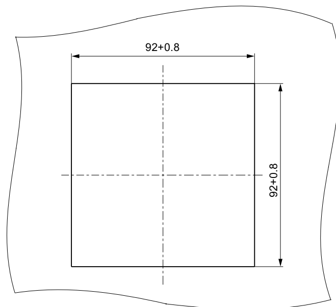
Bild 12-1 Schalttafelausschnitt
