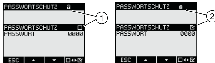
Bild 9-12 Geräteeinstellung "PASSWORTSCHUTZ"
