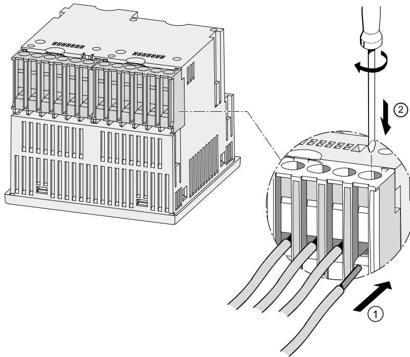
Bild 6-7 Anklemmen der Leitungen an der Schraubklemme
