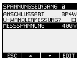
Bild 7-7 Geräteeinstellung "MESSSPANNUNG"
