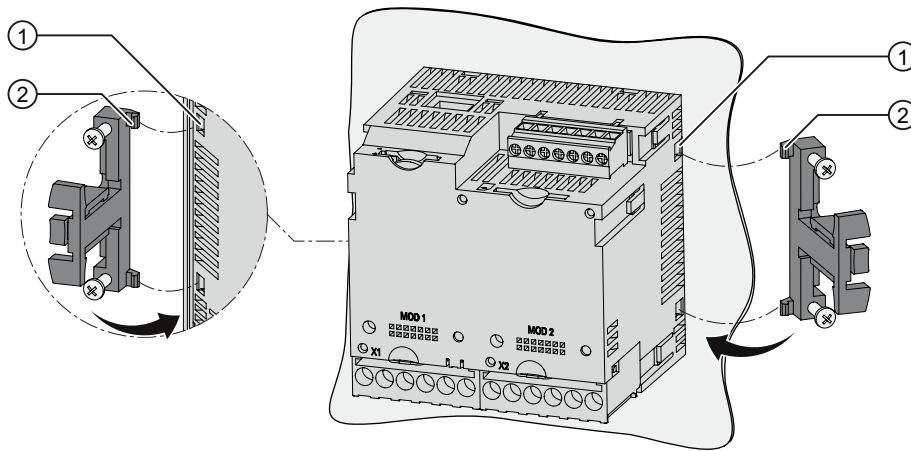
Montageschritt B
