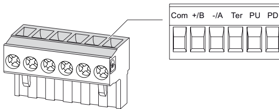
Bild 6-24 Klemmenbelegung
