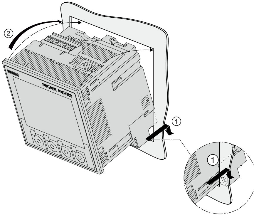
Bild 5-3 Montageschritt A, Gerät mit Ringkabelschuhanschlüssen
