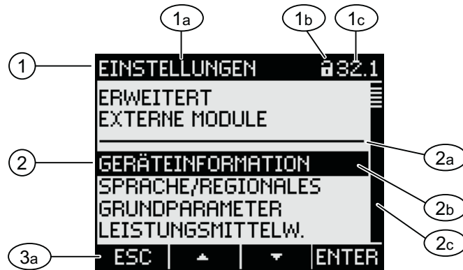
Bild 8-10 Anzeige "EINSTELLUNGEN"
