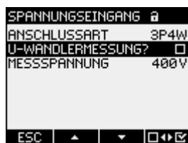
Bild 7-5 Geräteeinstellung "U-WANDLERMESSUNG"
