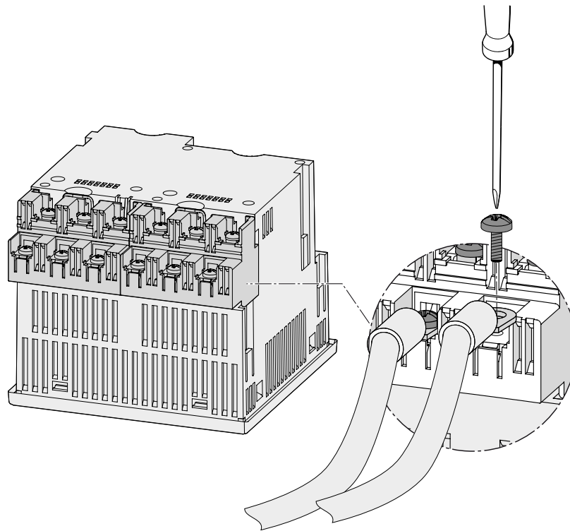
Bild 6-8 Anklemmen der Leitungen am Ringkabelschuhanschluss
