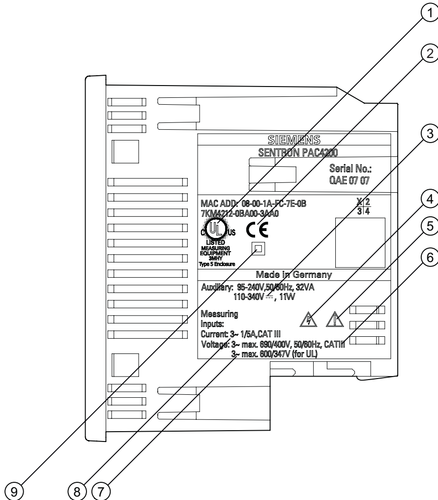
Bild 11-1 Gerätebeschriftung
