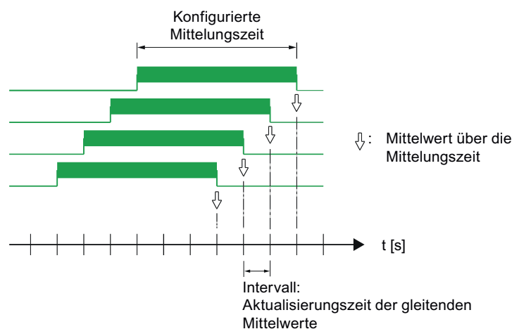
Bild 3-1 Gleitender Mittelwert
