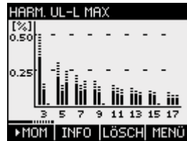
Bild 3-5 Momentanwerte und Maxima der Harmonischen der Spannung L-L, bezogen auf die Grundschiwingung
