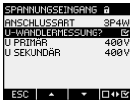
Bild 7-6 Geräteeinstellung "U-WANDLERMESSUNG?"
