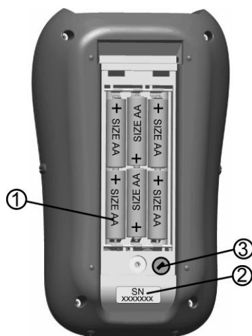
Bild 3.4: Batteriefach
