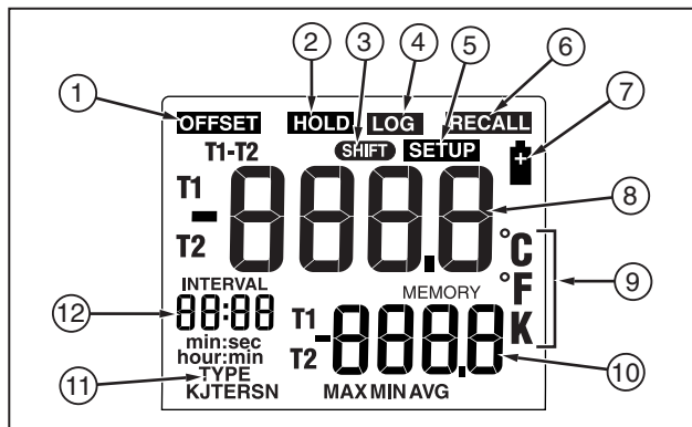
Abbildung 2. Anzeigeelemente
