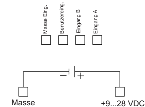
Bild 6.1: Anschlussklemmen
