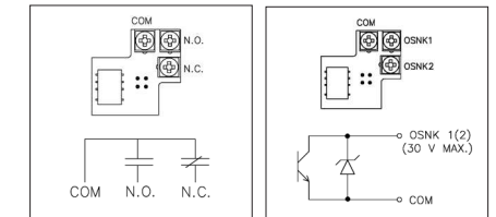
Relais Ausgangskarte
