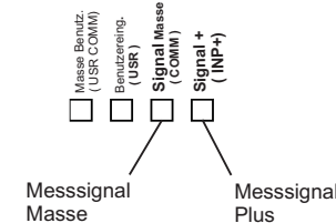
Bild 5.4: Anschlussklemmen und Karte
