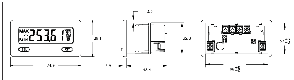
Bild 4.3: Abmessungen und Schalttafelausschnitt (Angaben in mm)
