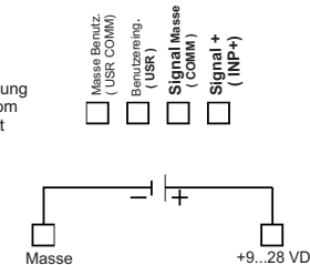
Bild 5.1: Anschlussklemmen
