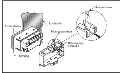
Bild 5.1: Montage
