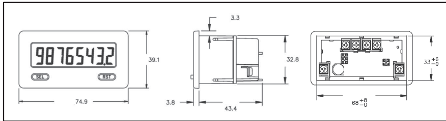
Bild 5.3: Abmessungen und Schalttafel ausschnitt (Angaben in mm)
