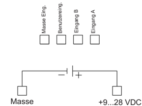
Bild 6.1: Anschlussklemmen
