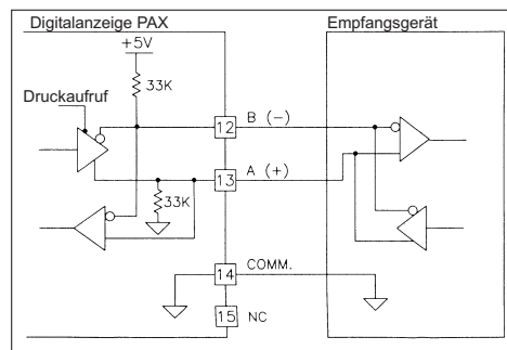
Bild 1.3: RS485-Schnittstelle PAXCDC10
