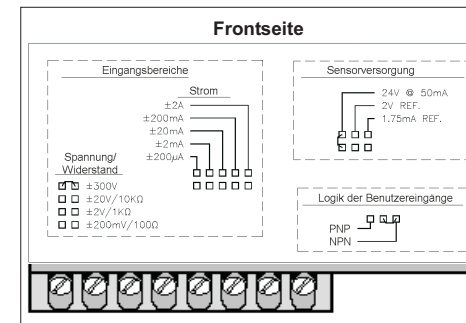
Bild 7.1: Jumper Einstellungen
