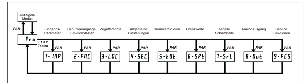
Bild 8.1: Das Programm-Menü
