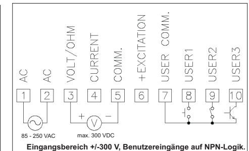
Bild 7.3: Anschlussbeispiel 1: Spannungssignal
