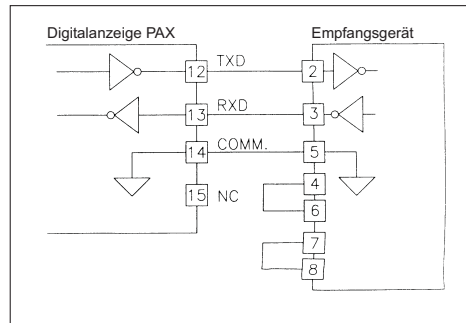
Bild 1.5: RS232-Schnittstelle PAXCDC20
