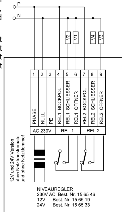
V1..V4 Verbraucher
