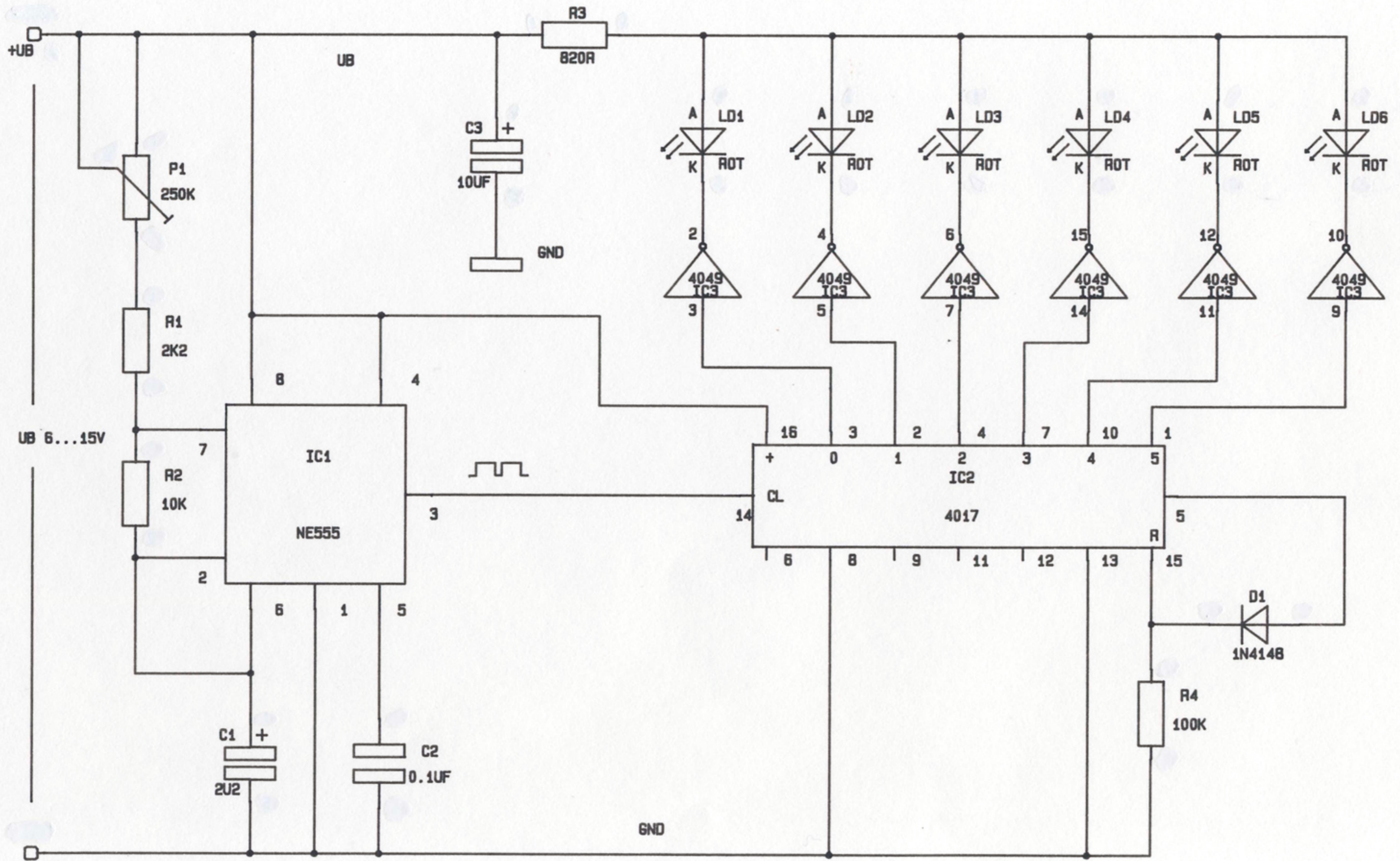
190128 6-Kanal-Lauflicht
