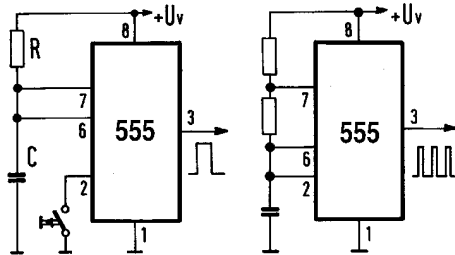
Bild 3: Beschaltung für den monostabilen (links) und astabilen Betrieb (rechts).
