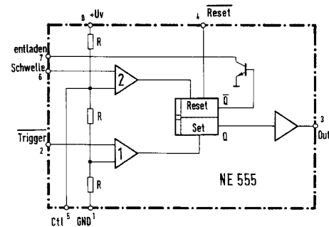
Bild 2: Innenbeschaltung des 555er.
