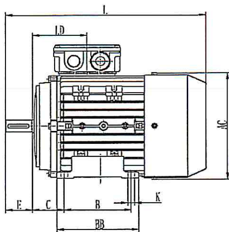
Anbaumaße, mm
