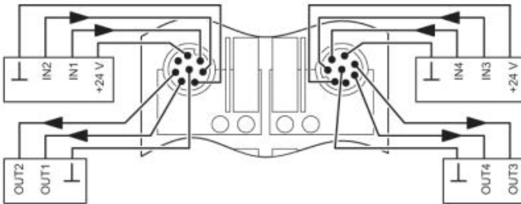
Anschlusszeichnung
