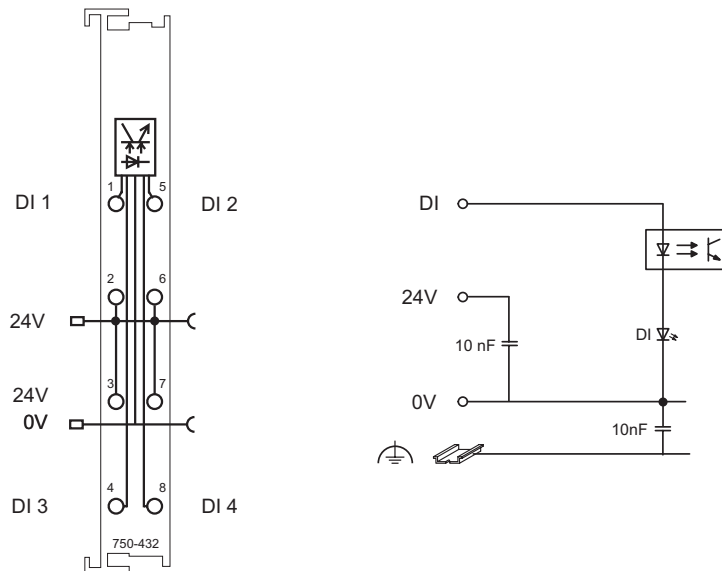
Abb. 2.1.1-3: 4-Kanal Digital Eingangsklemme 750-432
