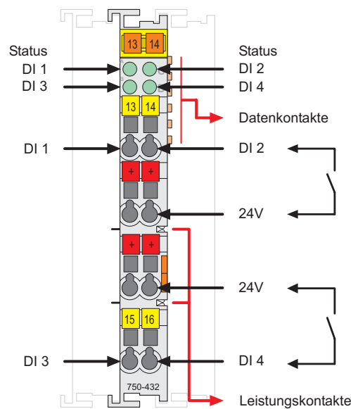
Abb. 2.1.1-1: 4-Kanal Digital Eingangsklemme 750-432
