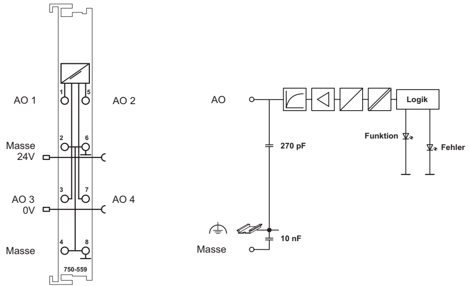
Abb. 2.1.1-3: 4-Kanal Analog Ausgangsklemme 750-559
