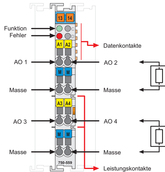
Abb. 2.1.1-1: 4-Kanal Analog Ausgangsklemme 750-559
