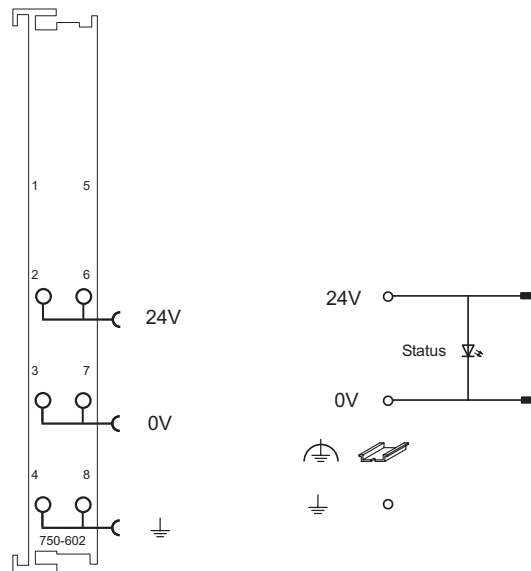
Abb. 2.1.1-3: Potentialeinspeiseklemme 750-602
