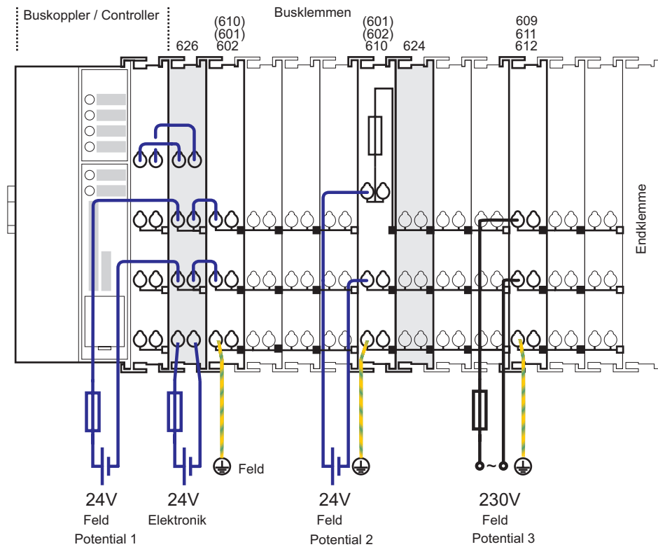
Abb. 2.1.1-4: Einspeisekonzept
