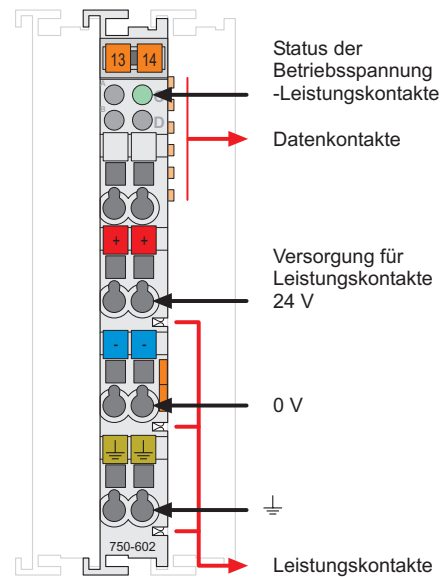
Abb. 2.1.1-1: Potentialeinspeiseklemme 750-602
