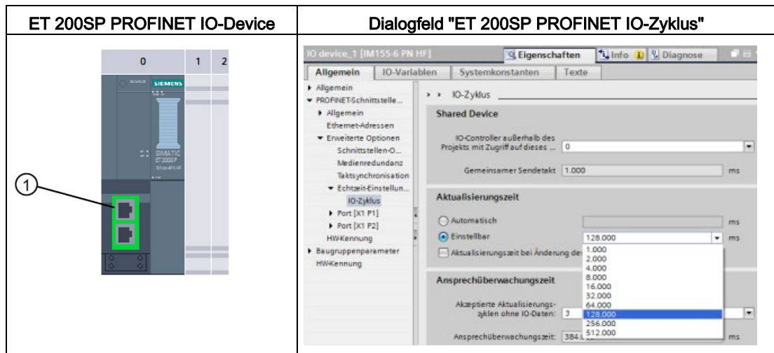
① PROFINET-Port
