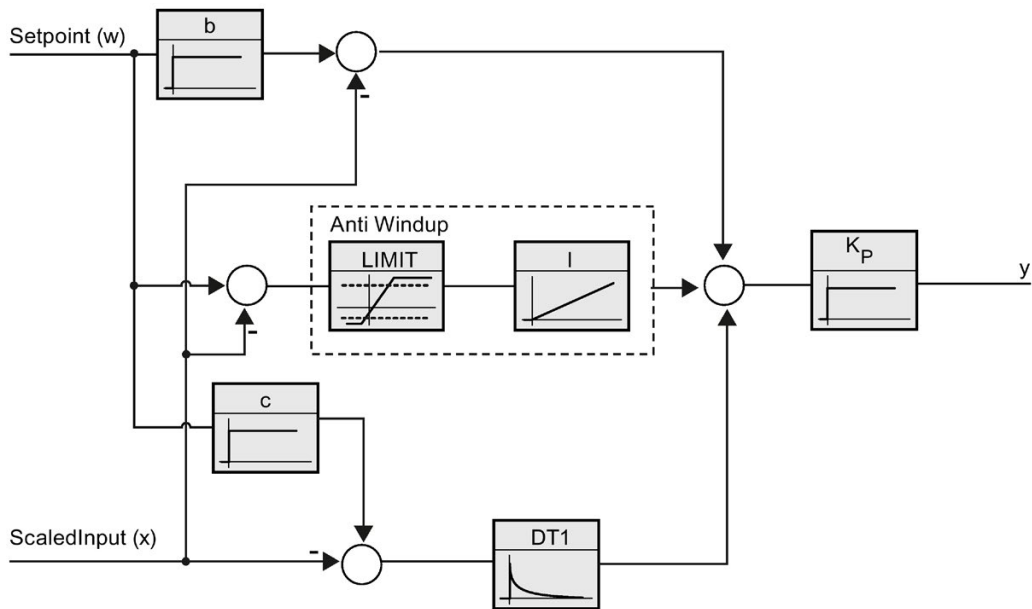
Bild 10-2 Funktionsweise des Reglers PID_Compact als PIDT1-Regler mit Anti-Windup
