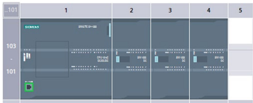
Bild 6-1 Gerätekonfiguration für Maximalausbau mit drei Signalmodulen
