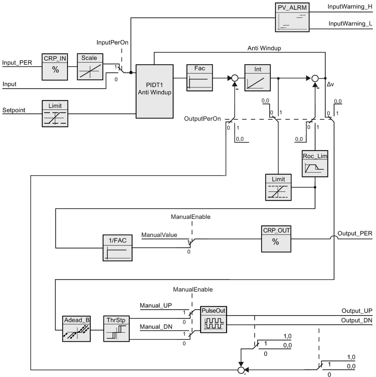
Bild 10-4 Funktionsweise des Reglers PID_3Step ohne Positionsrückmeldung
