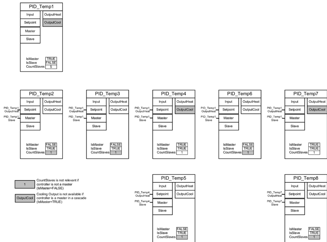
Bild 10-8 PID_Temp_Cascading_communication_connection
