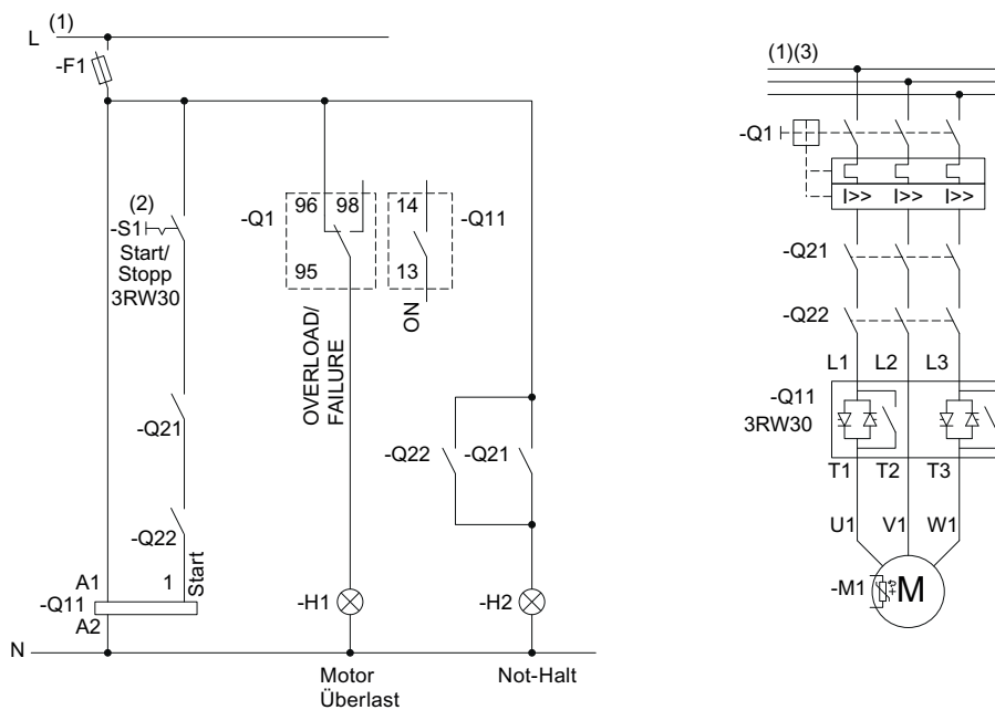
Bild 15-24 Verdrahtung Steuerstromkreis und Hauptstromkreis 3RW30
