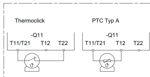
Bild 15-1 Optionale Thermistormotorschutz-Auswertung
