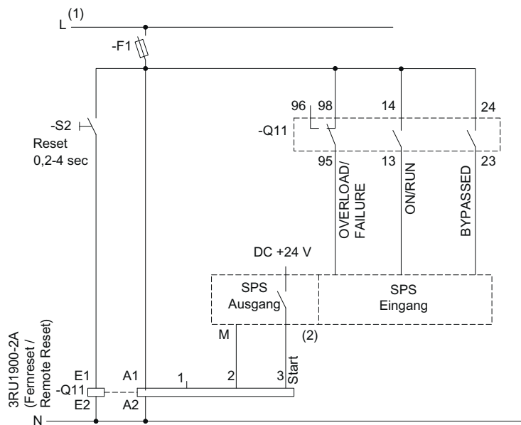
Bild 15-13 Verdrahtung Steuerstromkreis 3RW40 5 - 3RW40 7
