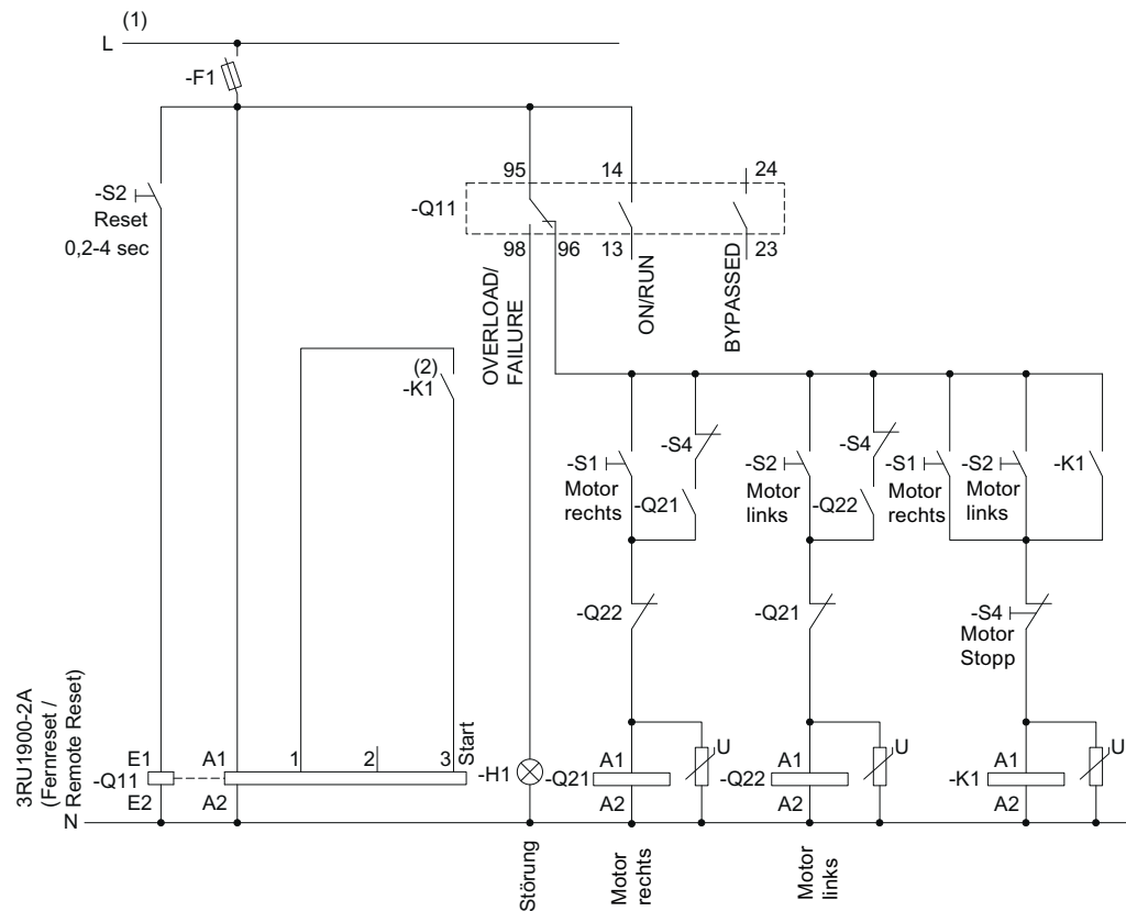
Bild 15-19 Verdrahtung Steuerstromkreis 3RW40 5 - 3RW40 7
