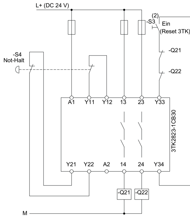
Bild 15-23 Verdrahtung Steuerstromkreis Not-Halt Sicherheitsschaltgerät 3TK28
