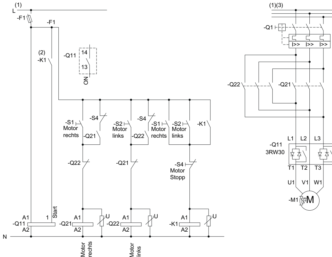
Bild 15-17 Verdrahtung Steuerstromkreis und Hauptstromkreis 3RW30
