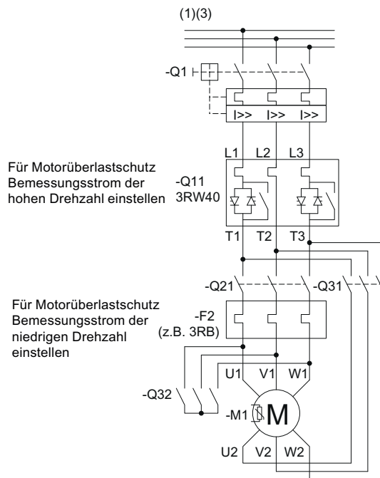
Bild 15-35 Verdrahtung Hauptstromkreis 3RW40 5 - 3RW40 7
