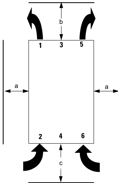
Bild 7-1 Abstand zu anderen Geräten
