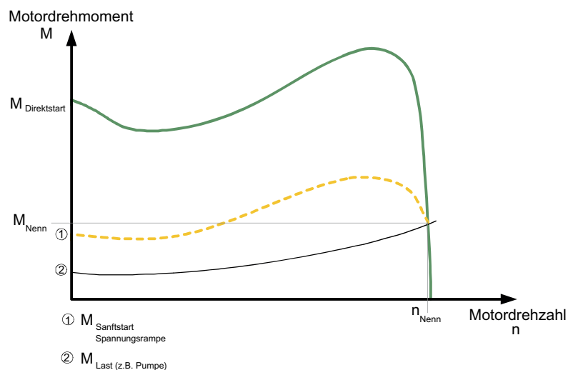
Bild 3-4 Reduziertes Drehmomentverhalten des Drehstrom-Asynchronmotors im Anlauf mit SIRIUS Sanftstarter 3RW30 oder 3RW40
