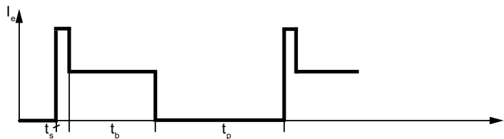
Bild 11-1 Einschaltdauer ED
