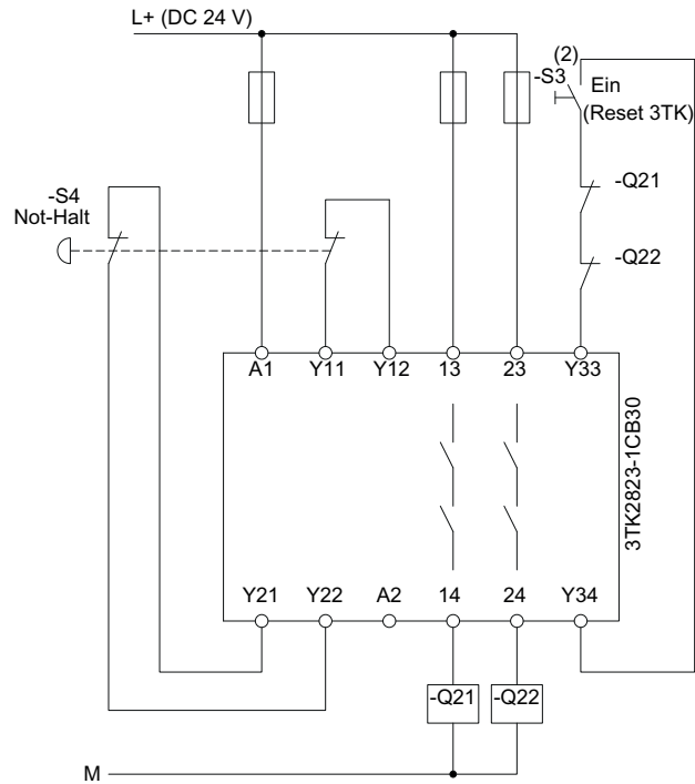
Bild 15-27 Verdrahtung Steuerstromkreis Not-Halt Sicherheitschaltgerät 3TK28
