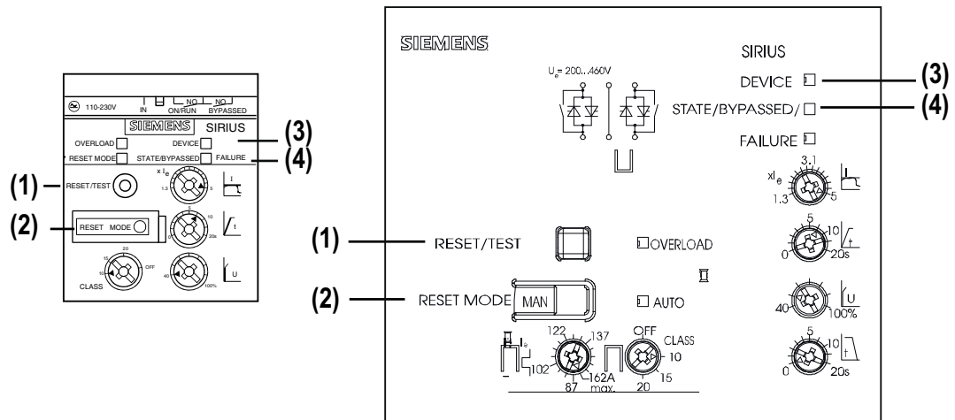
Bild 12-1 Tasten/LED-Übersicht 3RW40 2 - 3RW40 4 und 3RW40 5 - 3RW40 7
