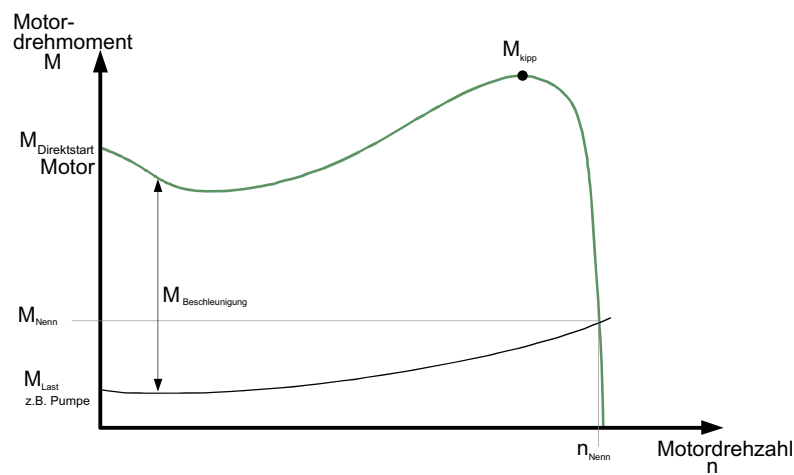
Bild 3-2 Typisches Anlaufdrehmomentverhalten eines 3-Phasen-Asynchronmotors
