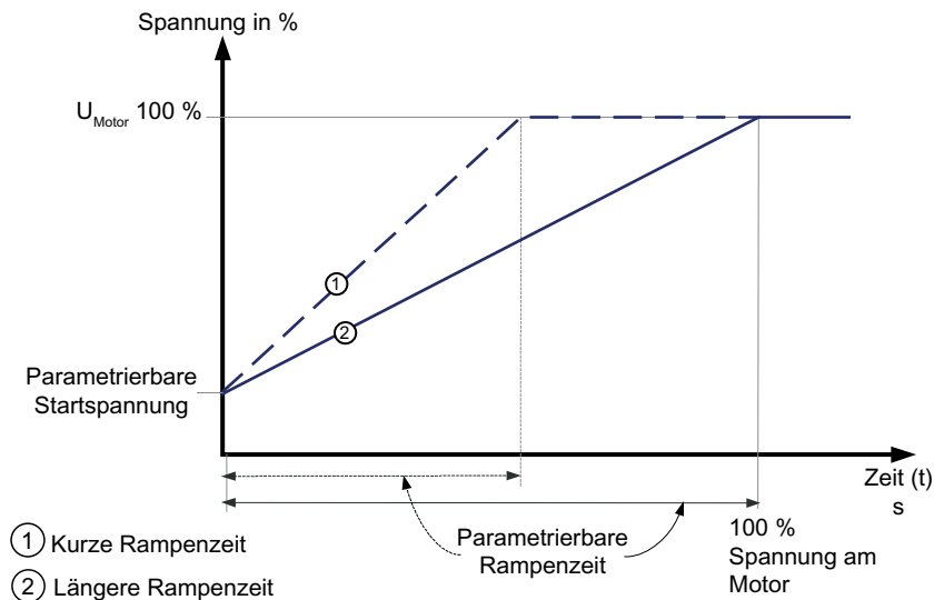
Bild 5-1 Funktionsprinzip Spannungsrampe
