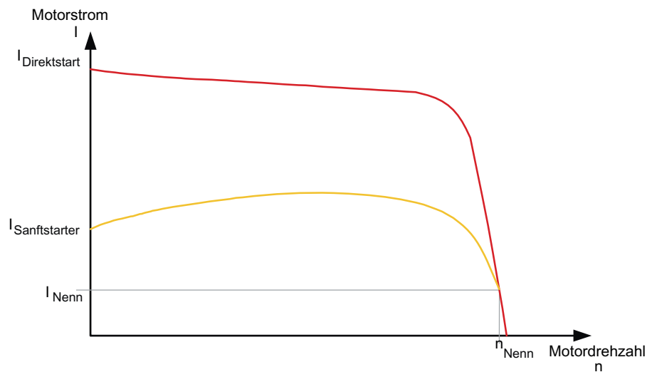
Bild 3-3 Reduziertes Stromverhalten des Drehstrom-Asynchronmotors im Anlauf mit SIRIUS Sanftstarter 3RW30 oder 3RW40
