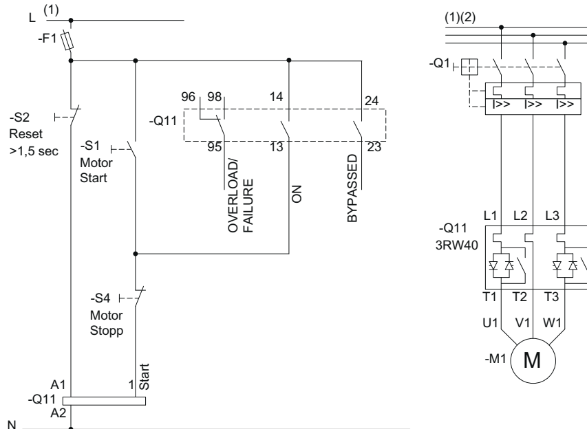
Bild 15-3 Verdrahtung Steuerstromkreis 3RW40 2 - 3RW40 4 und Hauptstromkreis 3RW40 2 - 3RW40 7
