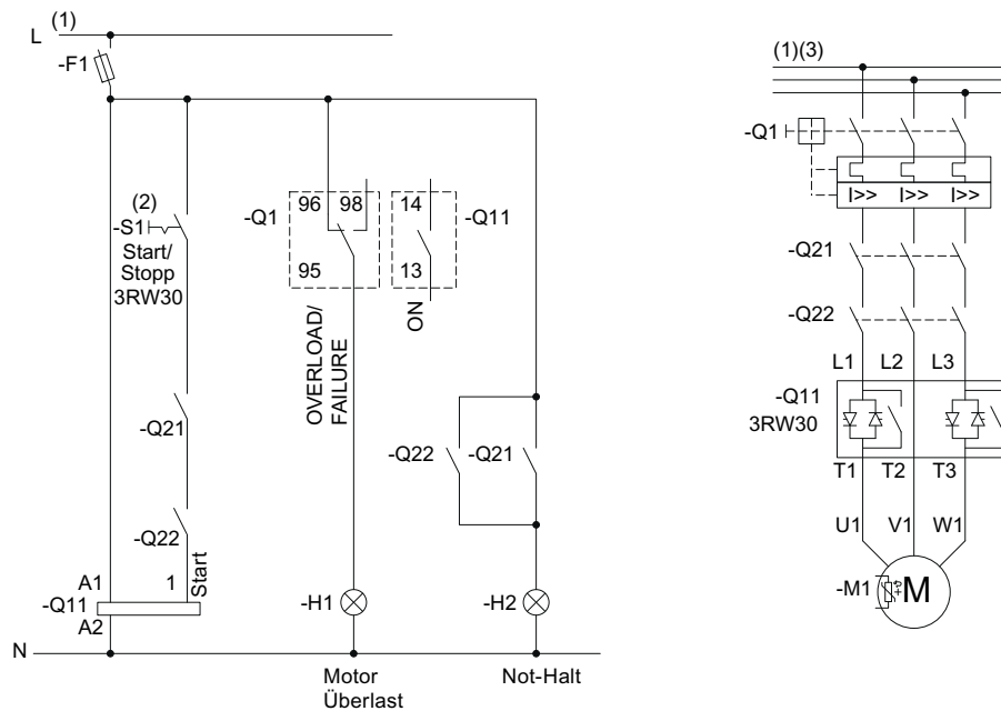
Bild 15-24 Verdrahtung Steuerstromkreis und Hauptstromkreis 3RW30
