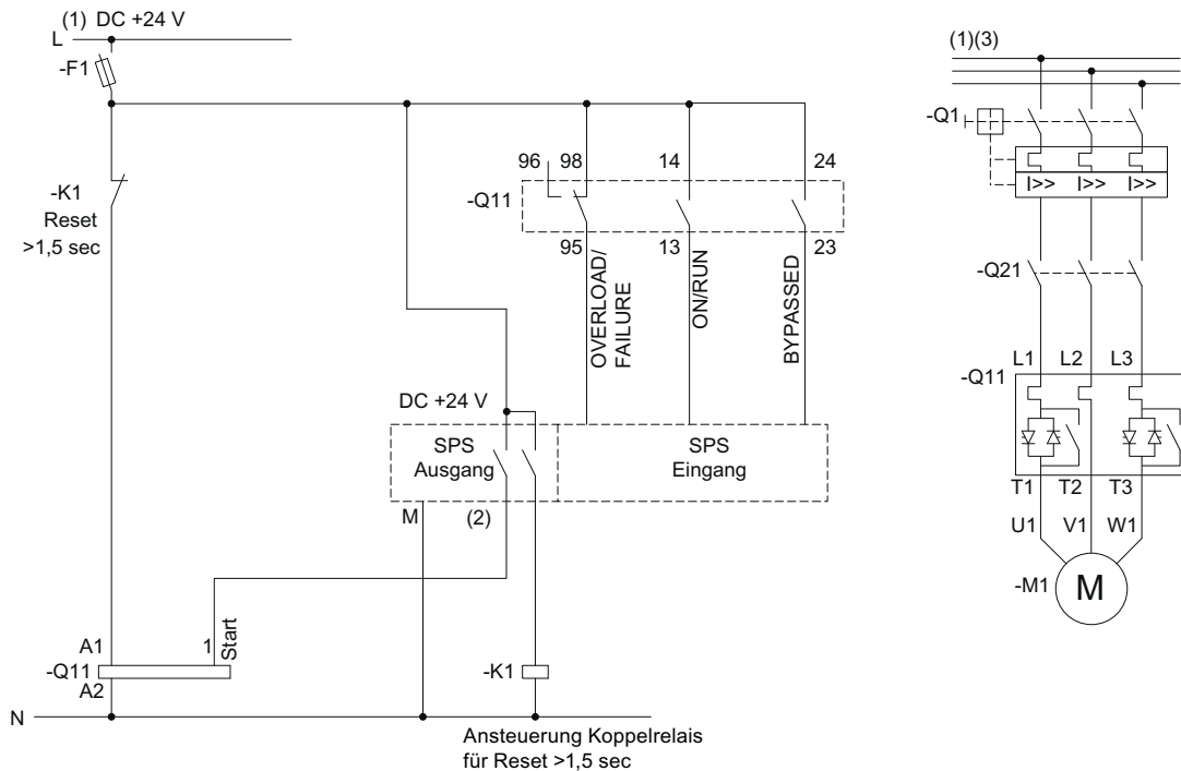
Bild 15-12 Verdrahtung Steuerstromkreis 3RW40 2 - 3RW40 4 (mit 24 V Steuerspannung) und Hauptstromkreis 3RW40 2 - 3RW40 7
