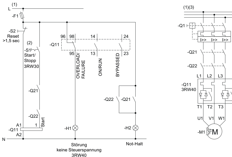
Bild 15-26 Verdrahtung Steuerstromkreis 3RW40 2 - 3RW40 4 und Hauptstromkreis 3RW402 bis 3RW40 7
