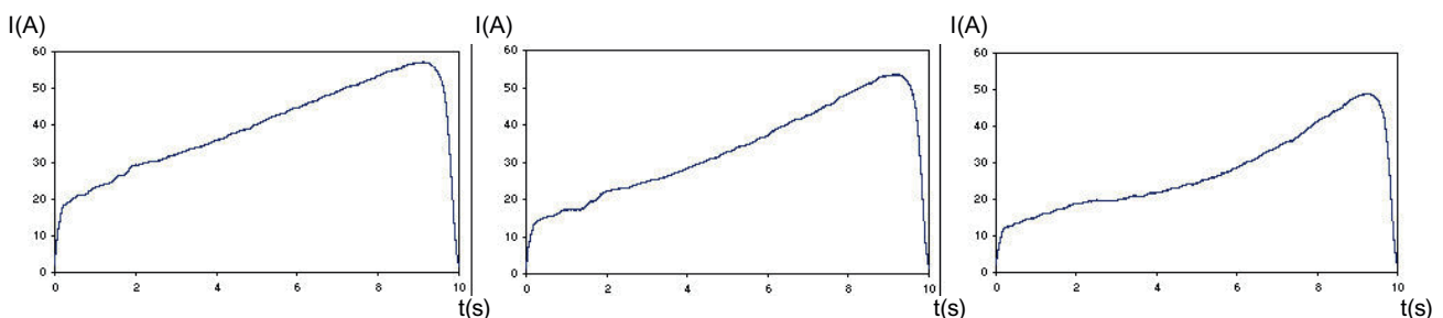
Bild 3-7 Stromverlauf in den 3 Phasen ohne Gleichstromanteile durch das "Polarity Balancing"-Ansteuerungsverfahren
