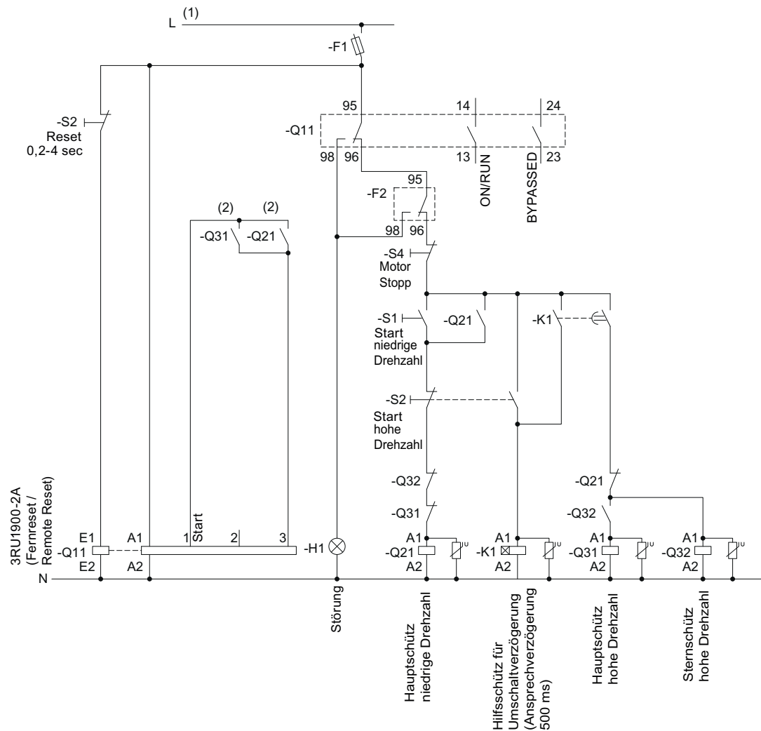
Bild 15-34 Verdrahtung Steuerstromkreis 3RW40 5 - 3RW40 7
