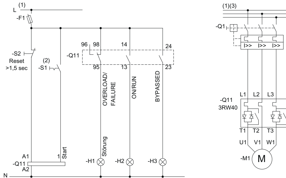
Bild 15-6 Verdrahtung Steuerstromkreis 3RW40 2 - 3RW40 4 und Hauptstromkreis 3RW40 2 - 3RW40 7
