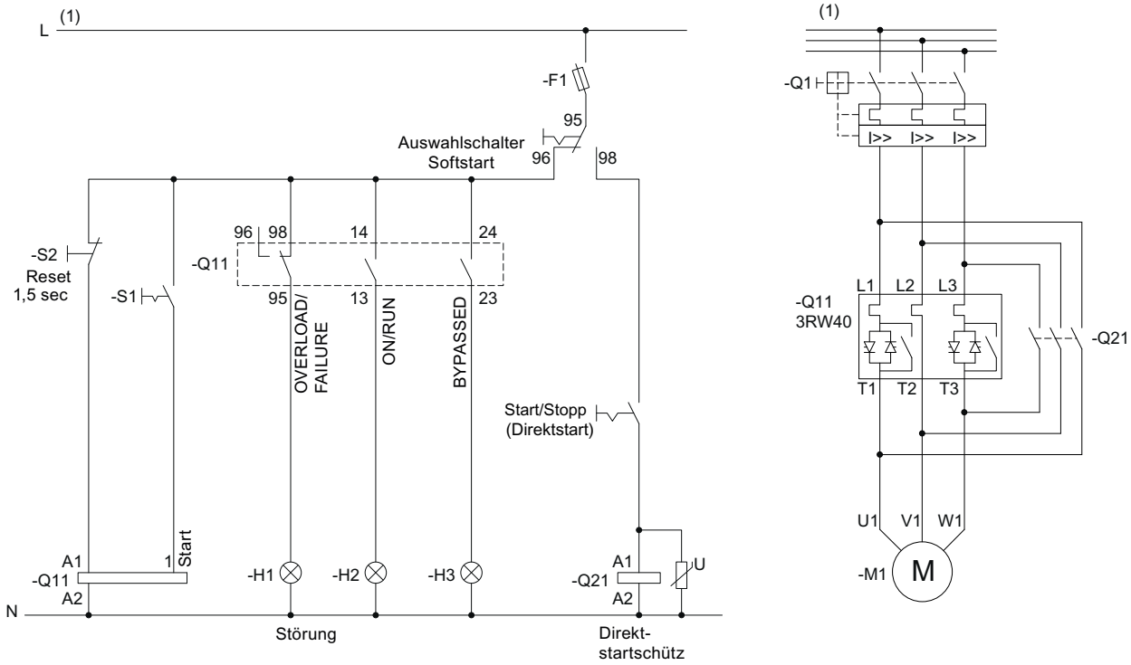
Bild 15-30 Verdrahtung Steuerstromkreis 3RW40 2 - 3RW40 4 und Hauptstromkreis 3RW40 2 bis 3RW40 7
