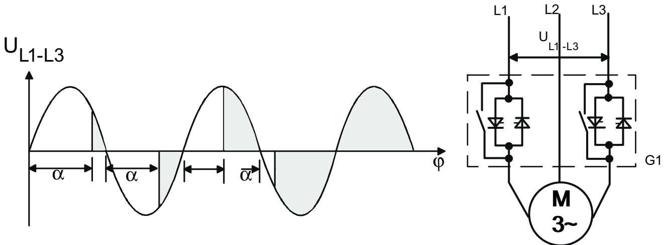
Bild 3-5 Phasenanschnittsteuerung und schematischer Aufbau eines 2-phasig gesteuerten Sanftstarters mit integrierten Bypasskontakten
