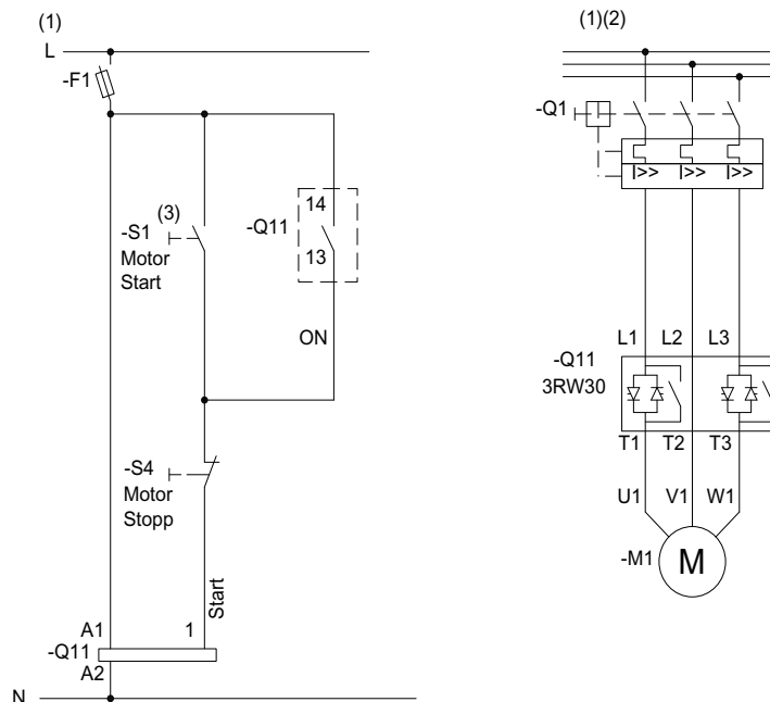
Bild 15-2 Verdrahtung Steuerstromkreis und Hauptstromkreis 3RW30
