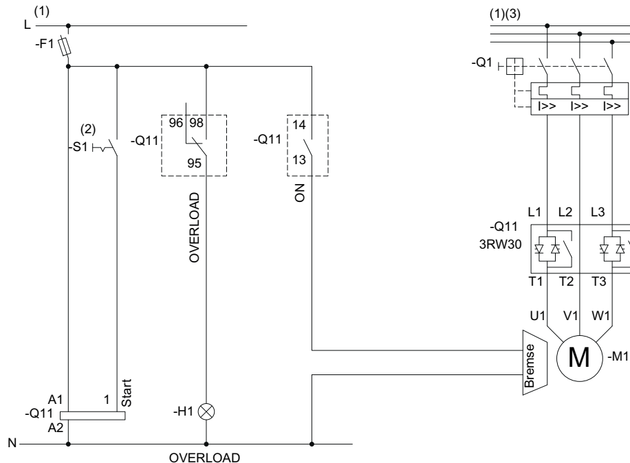
Bild 15-20 Verdrahtung Steuerstromkreis und Hauptstromkreis 3RW30
