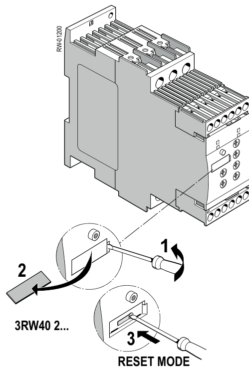
Bild 10-1 Taste zur Einstellung RESET MODE hinter Bezeichnungsschild
