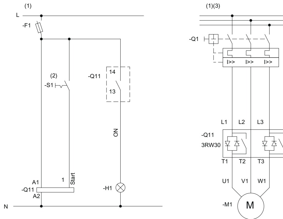
Bild 15-5 Verdrahtung Steuerstromkreis und Hauptstromkreis
