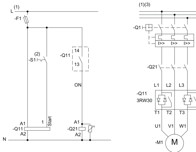
Bild 15-14 Verdrahtung Steuerstromkreis und Hauptstromkreis 3RW30
