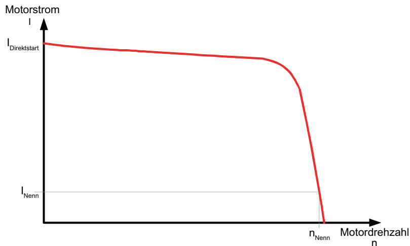
Bild 3-1 Typisches Anlaufstromverhalten eines 3-Phasen-Asynchronmotors
