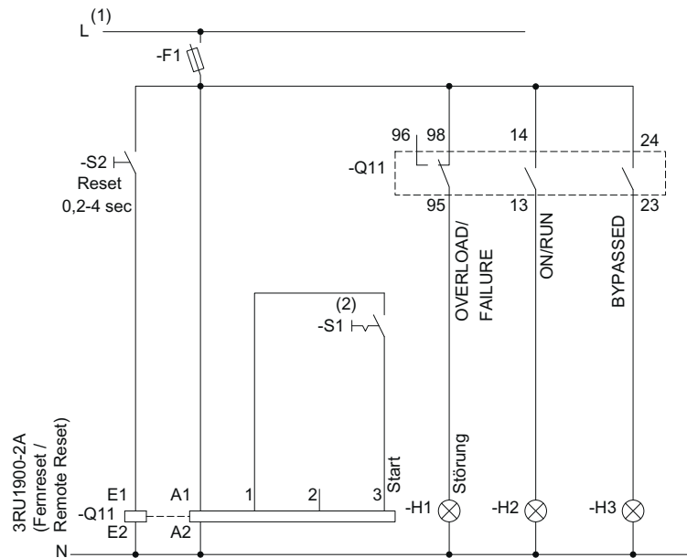
Bild 15-7 Verdrahtung Steuerstromkreis 3RW40 5 - 3RW40 7
