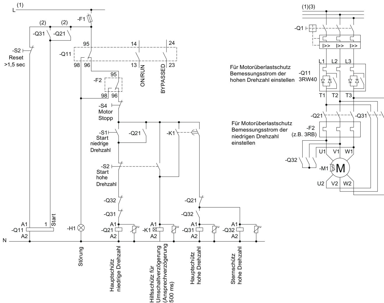
Bild 15-33 Verdrahtung Steuerstromkreis 3RW40 2 - 3RW40 4 und Hauptstromkreis 3RW40 2 bis 3RW40 7
