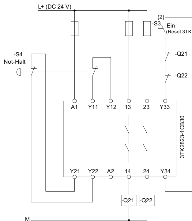
Bild 15-25 Verdrahtung Steuerstromkreis Not-Halt Sicherheitsschaltgerät 3TK28
