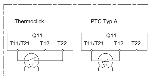
Bild 15-1 Optionale Thermistormotorschutz-Auswertung
