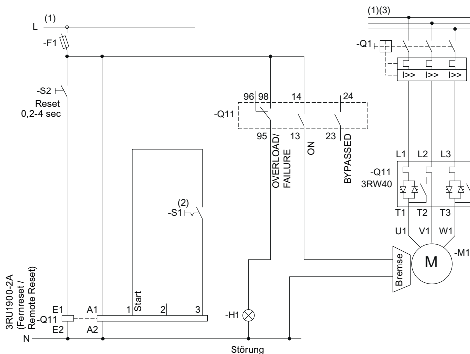
Bild 15-22 Verdrahtung Steuerstromkreis, Hauptstromkreis 3RW40 5 - 3RW40 7
