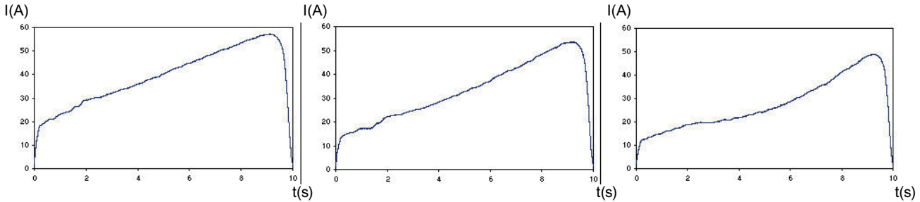
Bild 3-8 Unterschiedliche Höhe der Anlaufströme
