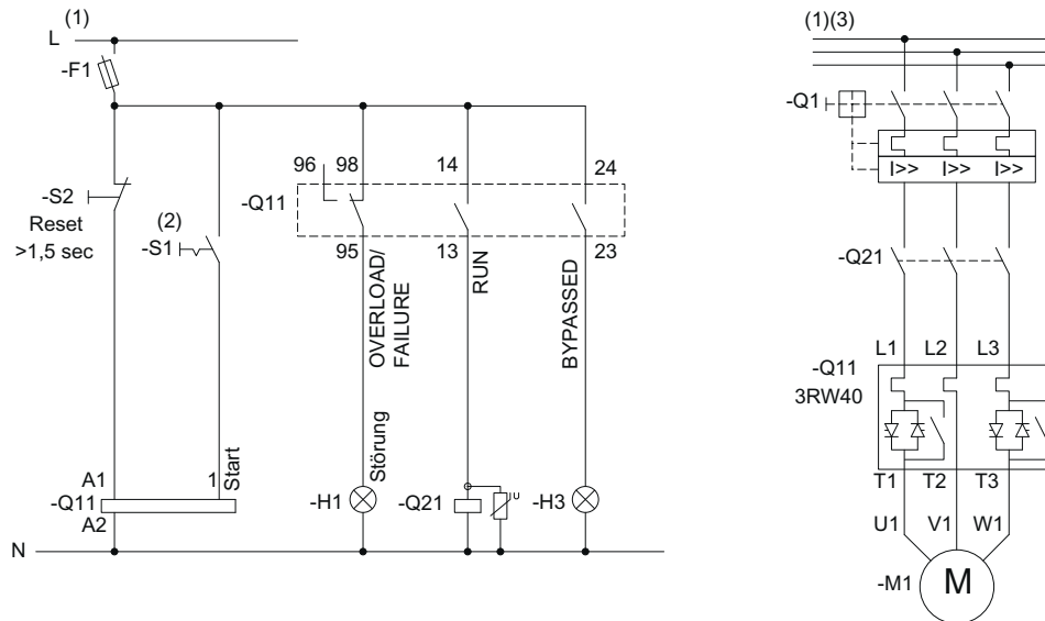
Bild 15-15 Verdrahtung Steuerstromkreis 3RW40 2 - 3RW40 4 und Hauptstromkreis 3RW40 2 - 3RW40 7
