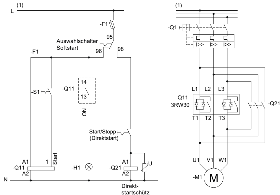
Bild 15-29 Verdrahtung Steuerstromkreis und Hauptstromkreis 3RW30
