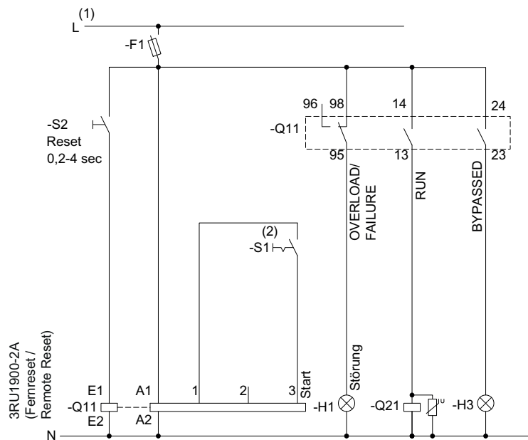
Bild 15-16 Verdrahtung Steuerstromkreis 3RW40 5 - 3RW40 7
