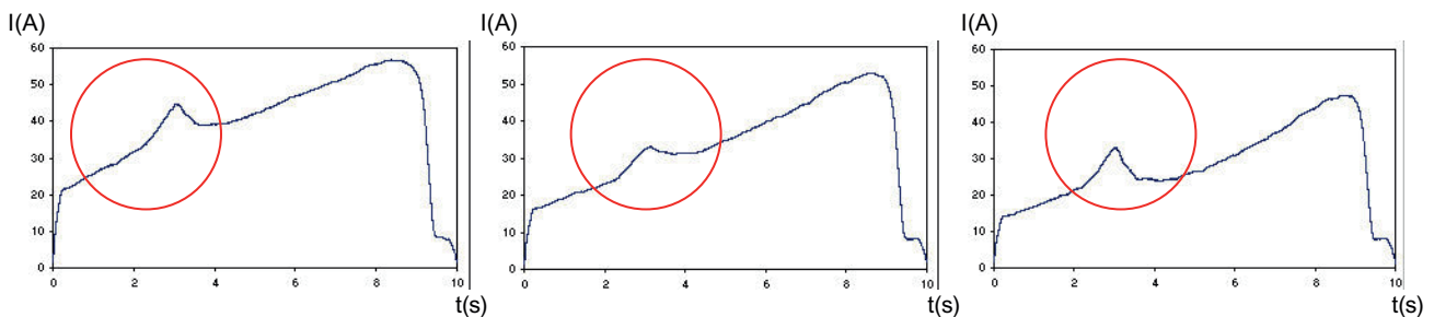
Bild 3-6 Stromverlauf und Auftreten der Gleichstromanteile in den 3 Phasen, ohne das "Polarity Balancing"-Ansteuerungsverfahren
