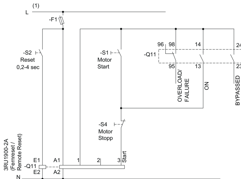
Bild 15-4 Verdrahtung Steuerstromkreis 3RW40 5 - 3RW40 7
