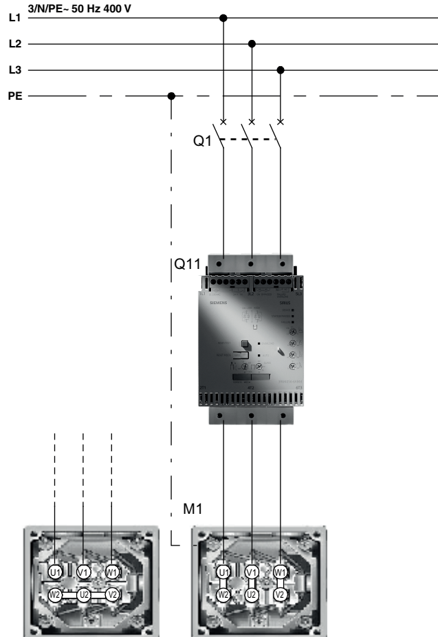
Bild 8-1 Prinzipschaltbild SIRIUS Sanftstarter 3RW40
