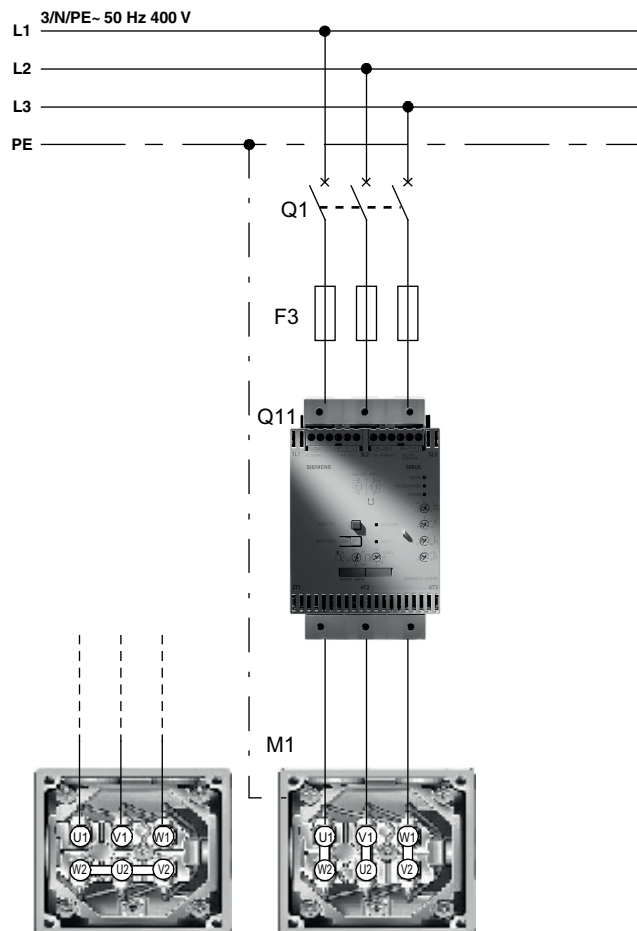
Bild 8-3 Prinzipschaltbild Abzweig mit Halbleiterschutzsicherungen
