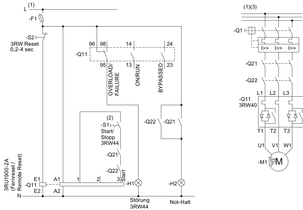
Bild 15-28 Verdrahtung Steuerstromkreis 3RW40 5 - 3RW40 7 und Hauptstromkreis 3RW40 2 bis 3RW40 7
