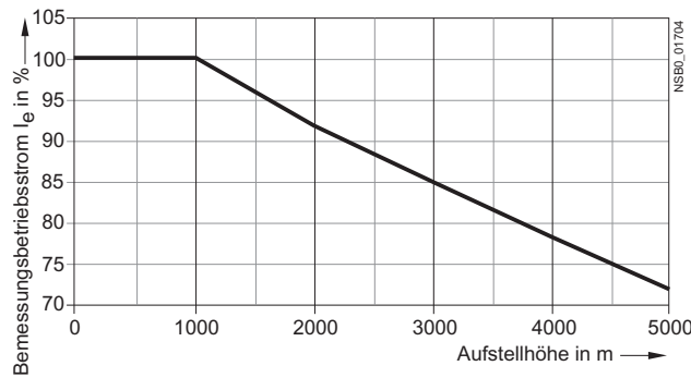
Bild 11-2 Reduzierung in Abhängigkeit von der Aufstellhöhe
