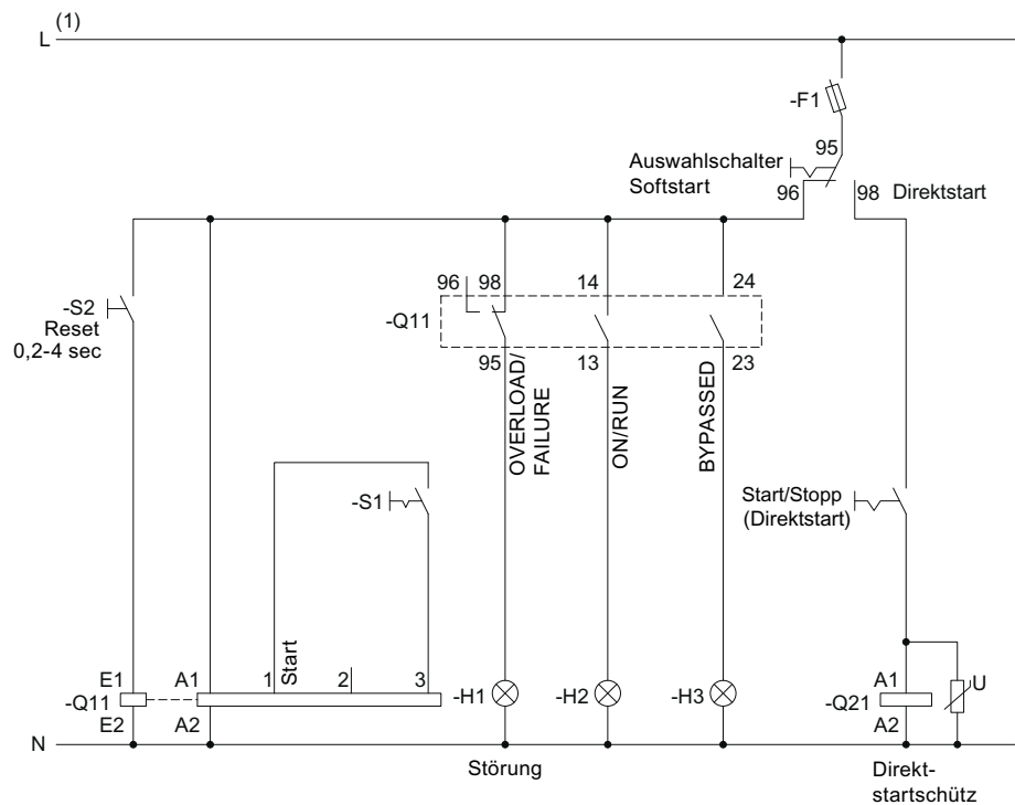
Bild 15-31 Verdrahtung Steuerstromkreis 3RW40 5 - 3RW40 7
