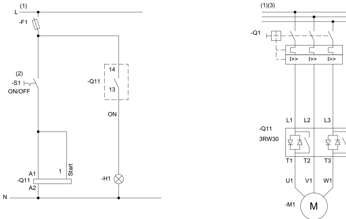
Bild 15-8 Verdrahtung Steuerstromkreis und Hauptstromkreis 3RW30
