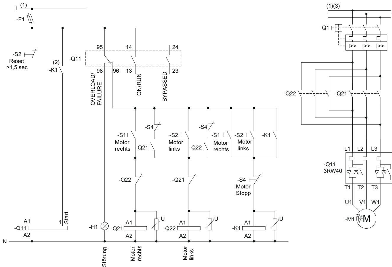
Bild 15-18 Verdrahtung Steuerstromkreis 3RW40 2 - 3RW40 5 und Hauptstromkreis 3RW40 2 - 3RW40 7
