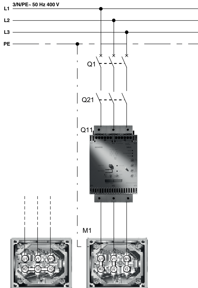
Bild 8-2 Prinzipschaltbild Abzweig mit optionalem Hauptschütz / Netzschütz
