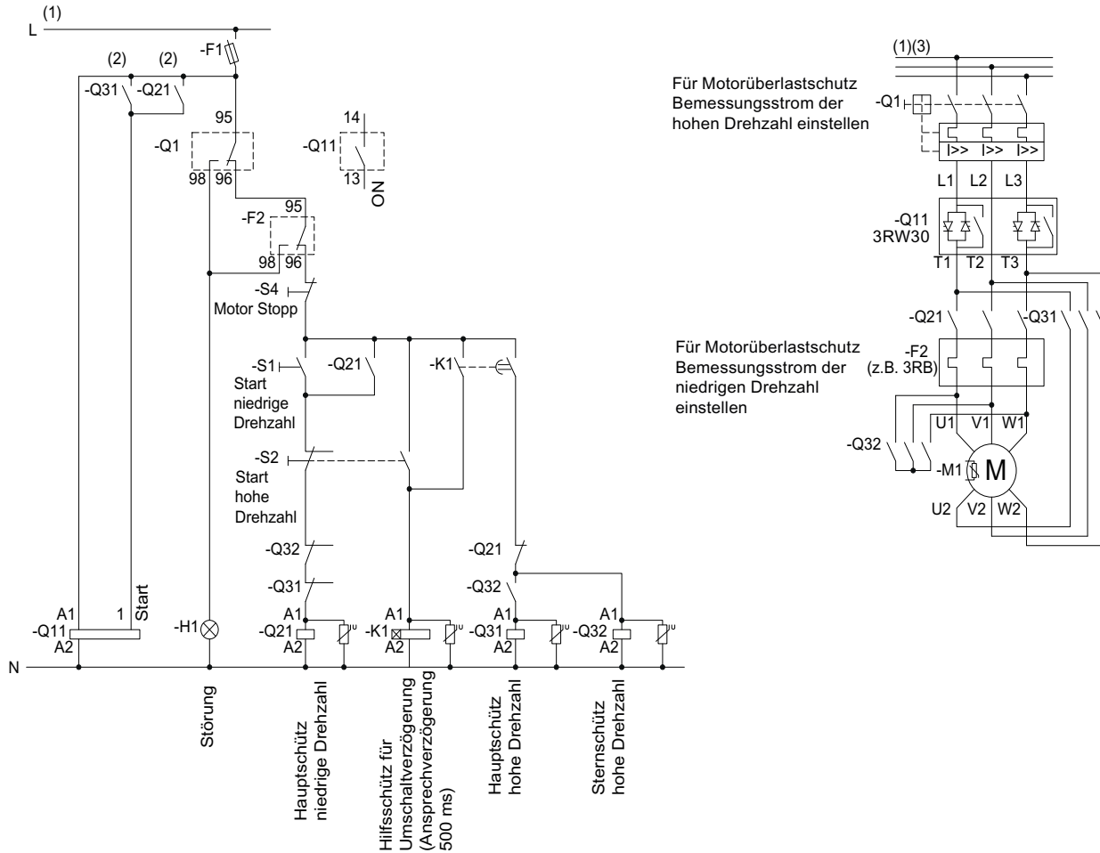
Bild 15-32 Verdrahtung Steuerstromkreis und Hauptstromkreis 3RW30
