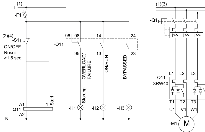
Bild 15-9 Verdrahtung Steuerstromkreis 3RW40 2 - 3RW40 4 und Hauptstromkreis 3RW40 2 - 3RW40 7
