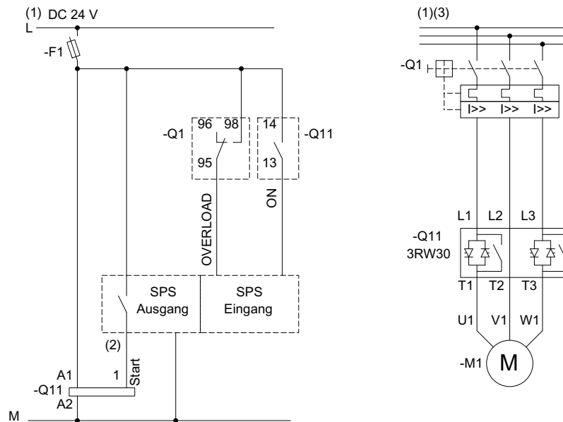
Bild 15-11 Verdrahtung Steuerstromkreis und Hauptstromkreis 3RW30
