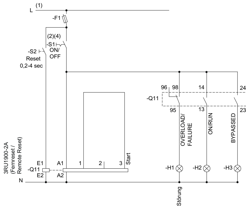
Bild 15-10 Verdrahtung Steuerstromkreis 3RW40 5 - 3RW40 7
