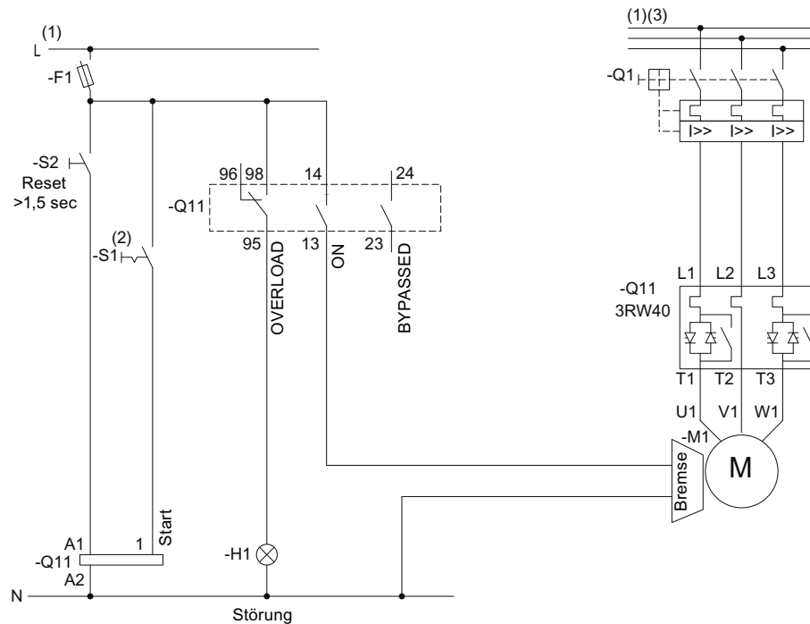
Bild 15-21 Verdrahtung Steuerstromkreis / Hauptstromkreis 3RW40 2 - 3RW40 4
