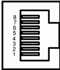
Bild 3-14 RJ45-Buchse
