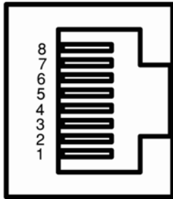
Bild 3-6 RJ45-Buchse
