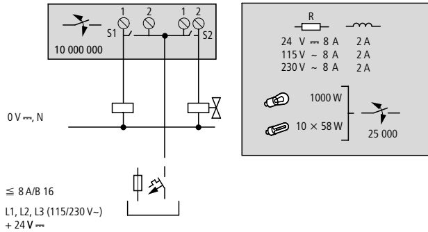
Abbildung 29: Relais-Ausgänge EASY2...-RE..
