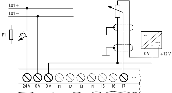
Abbildung 19: Sollwertgeber
