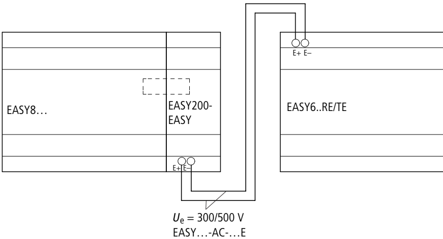
Abbildung 39: Dezentrale Erweiterungen an easy800 anschließen
