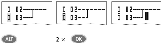
Abbildung 50: Kontakt I 13 von Schließer zu Öffner ändern
