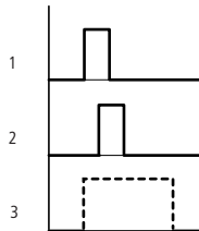
Abbildung 100: Wirkdiagramm PUT-Baustein
