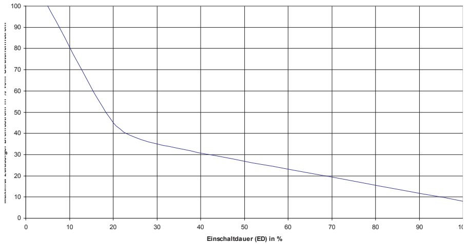
Belastungskurve für BR 230/400-30L (LP)
