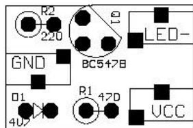
Fig. 2 Bestückungsplan
