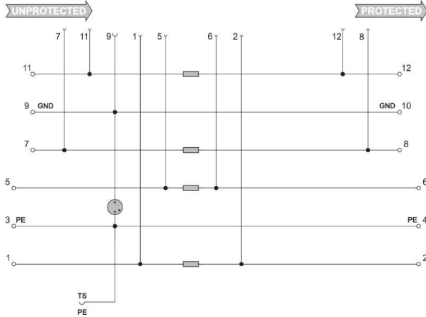
Prinzipialschaltbild
