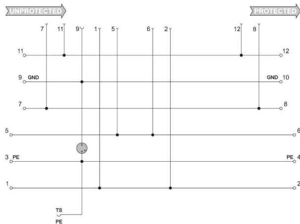
Prinzipschaltbild
